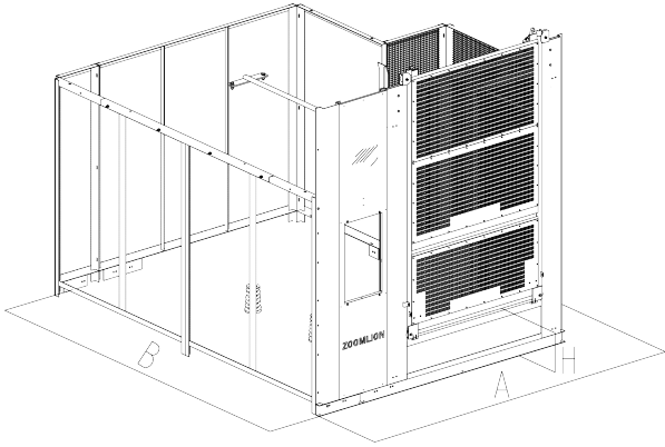
⑤ 右单笼带司机室围栏 enclosure for right cage with cab Ограждение для правой клетки с кабиной Sağdaki kabinli kafes muhafazası قفص فردي أيمن مع درابزين كابينة السائق
