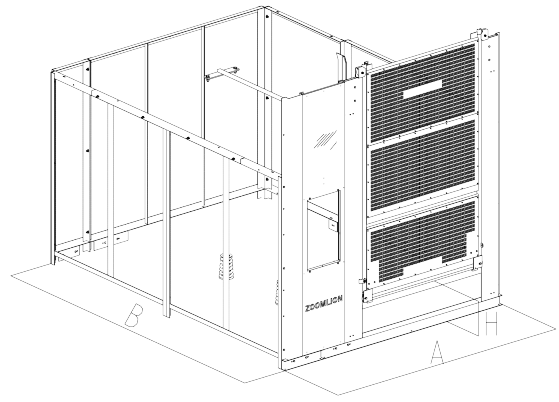
⑥ 右单笼不带司机室围栏 enclosure for right cage without cab Ограждение для правой клетки без кабины Sağdaki kabinsiz kafes muhafazası قفص فردي أيمن بدون درابزين كابينة السائق
