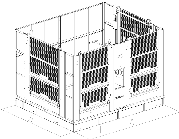
⑦ 带C门双笼围栏 enclosure for double cage with C-door Ограждение с двойной клеткой и C-образной дверью C kapılı çift kafesli çit سياج مزدوج القفص مزود بباب على شكل C
