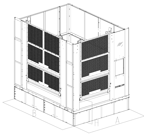
⑧ 带C门单笼围栏 enclosure for single cage with C-door Ограждение с одинарной клеткой и C-образной дверью C kapılı tek kafesli çit سياج قفص واحد مزود بباب على شكل C
